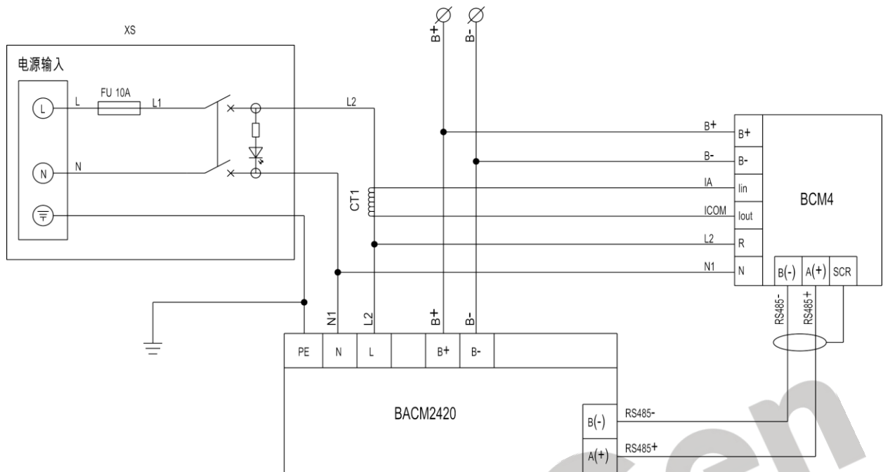
图 5 充电器和控制器内部接线图
